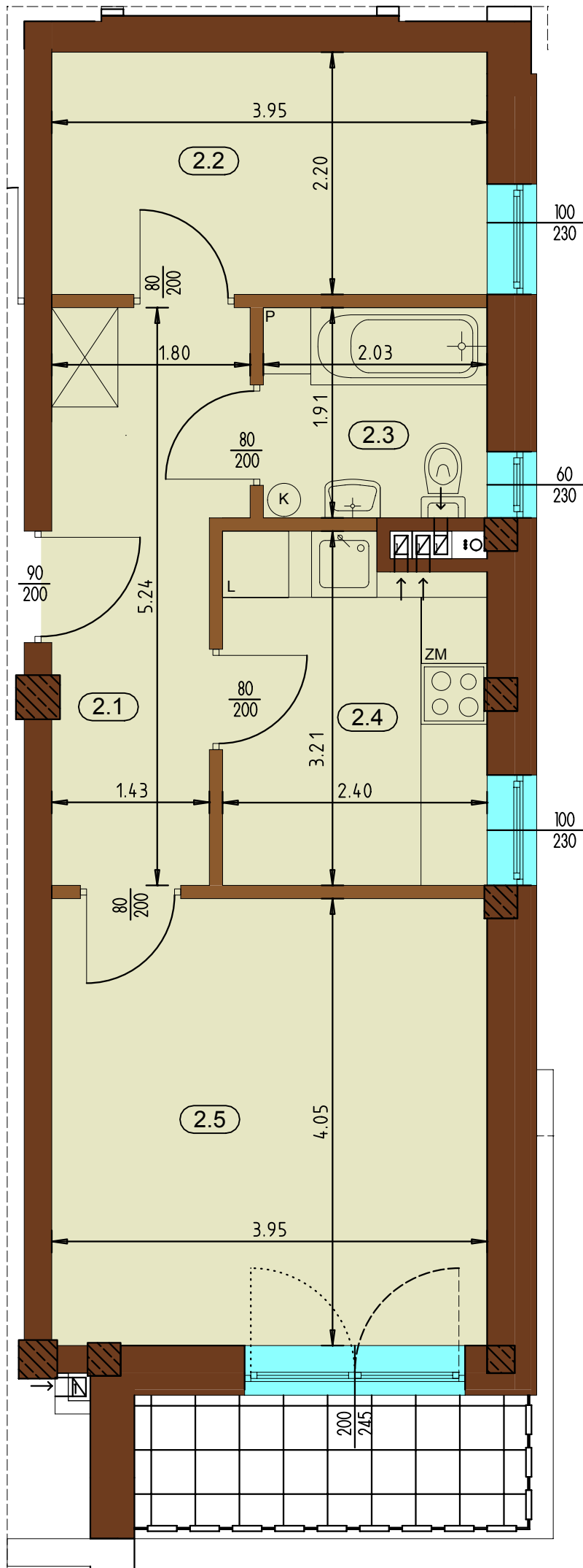
MIESZKANIE M-6 (PIĘTRO I) SKALA 1:50
