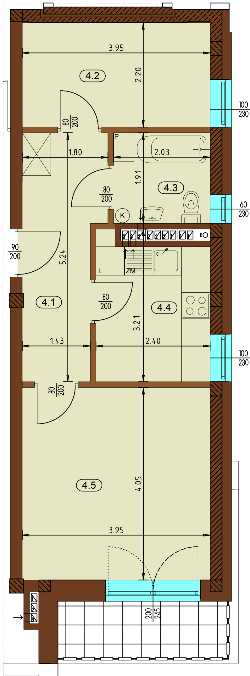
MIESZKANIE M-24 (PIĘTRO III) SKLALA 1:50
