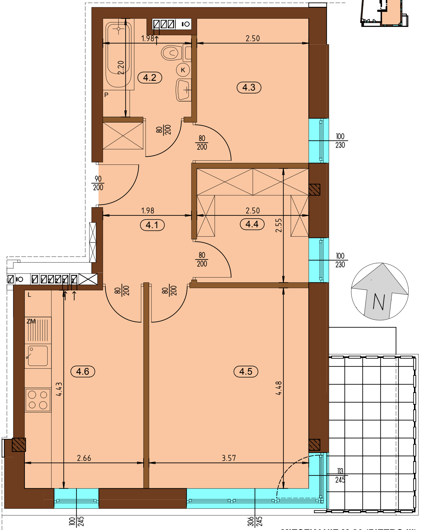
MIESZKANIE M-26 (PIĘTRO III) SKLALA 1:50
