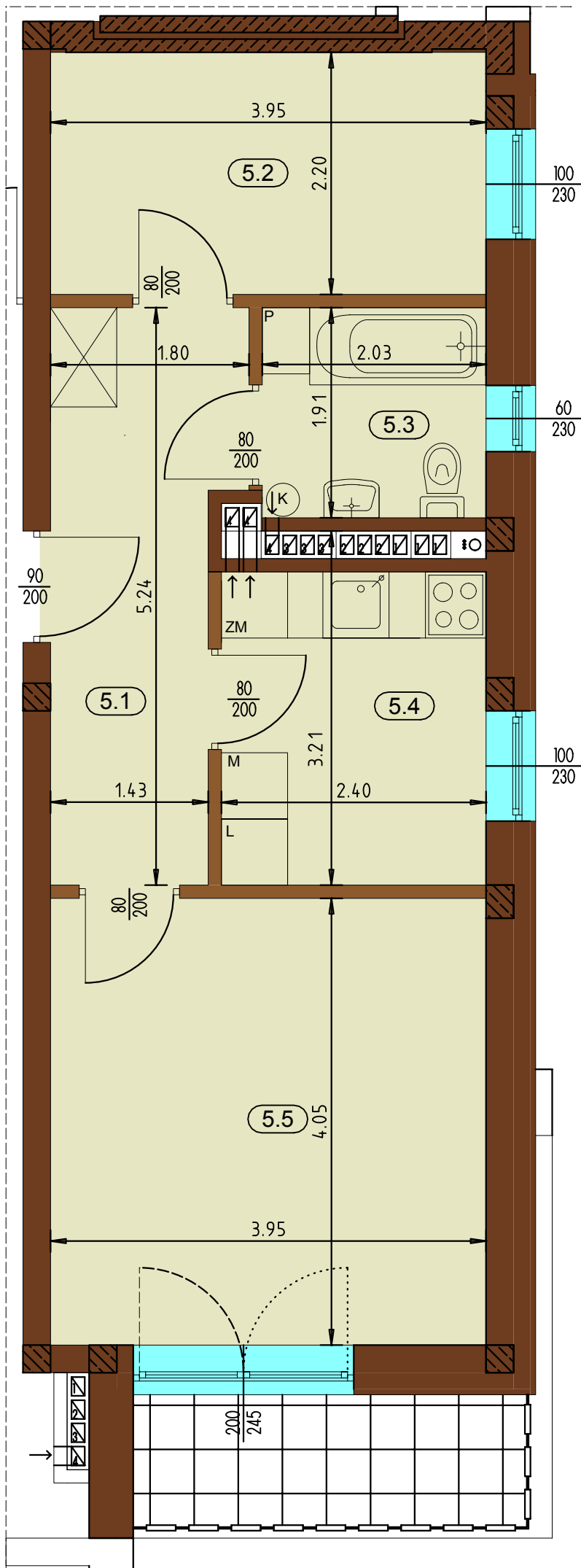
MIESZKANIE M-33 (PIĘTRO IV) SKLALA 1:50
