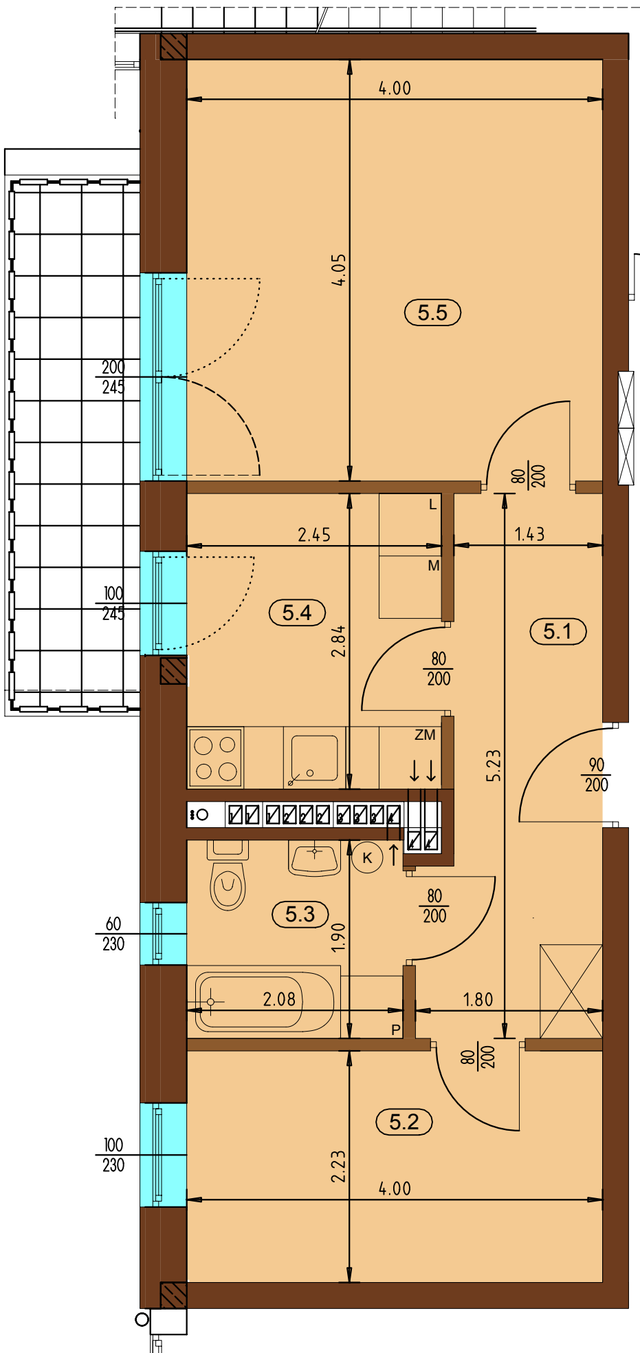
MIESZKANIE M-34 (PIĘTRO IV) SKLALA 1:50
